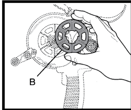
2. 12 mm巾のテープを使用する場合には、テープロールスペーサー〈B〉を本体に残す。18 mm巾のテープを使用する場合には、テープロールスペーサーを回転させて取り外します。
