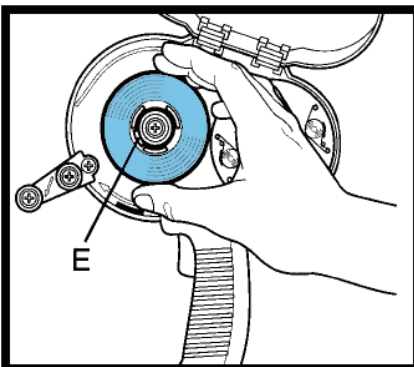
4. テープロールをハブの三本指の上に置いて、フック〈E〉がテープロールにきちんと上に出るまでテープを押さえてセットします。
