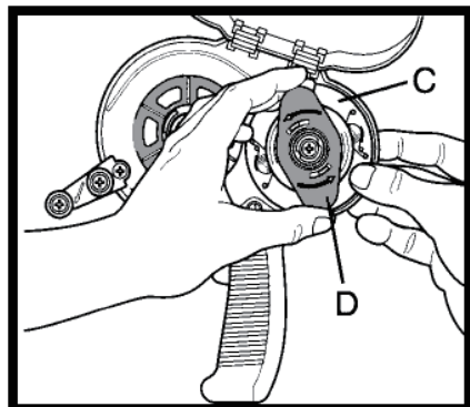
3. 巻き戻しハブ〈C〉を保体と一緒に挟む様に押さえて、ライナー保持器〈D〉を左回りに少し回転させてロックを外し、ロックが外れたら持ち上げてライナー保持器取り出します。
