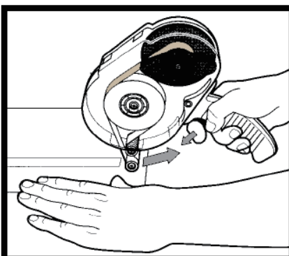
7. テープの転写を終わるには、終了位置で引き金を戻して、アプリケーターを少し上上げる様に手前に引っ張り粘着材を切り離します。尚、真上に引き上げると粘着材を綺麗に切り離す事が出来ません。
