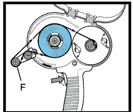
5. 図の様に引き金を押してテープのリーダーを〈F〉の位置で折り返してライナー保持器のスリットに入れて先端のテープ部分を本体に固定します。引き金を外して保持器を右側に回転させてテープの弛みを無くしてライナー保持器を元に戻してロックするまで回転させて固定し、12 mm巾の場合には、テープロールスペーサーも戻して本体カバーを閉じます。
