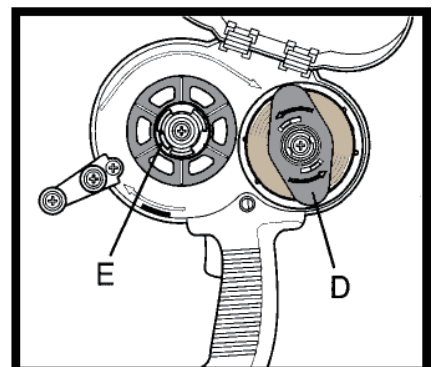
8. 使用を終了したテープを交換する場合には、ライナー保持器〈D〉を取り外して不要になったライナーを取り出します。テープの芯を取り出すには、フック〈E〉を内側に押さえて不要なテープ芯を取り出します。
